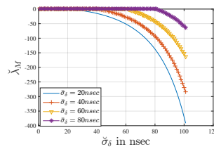
Fig. 3: \check{\lambda}_M v.s. \check{\sigma}_\delta for different \check{\sigma}_\delta .
